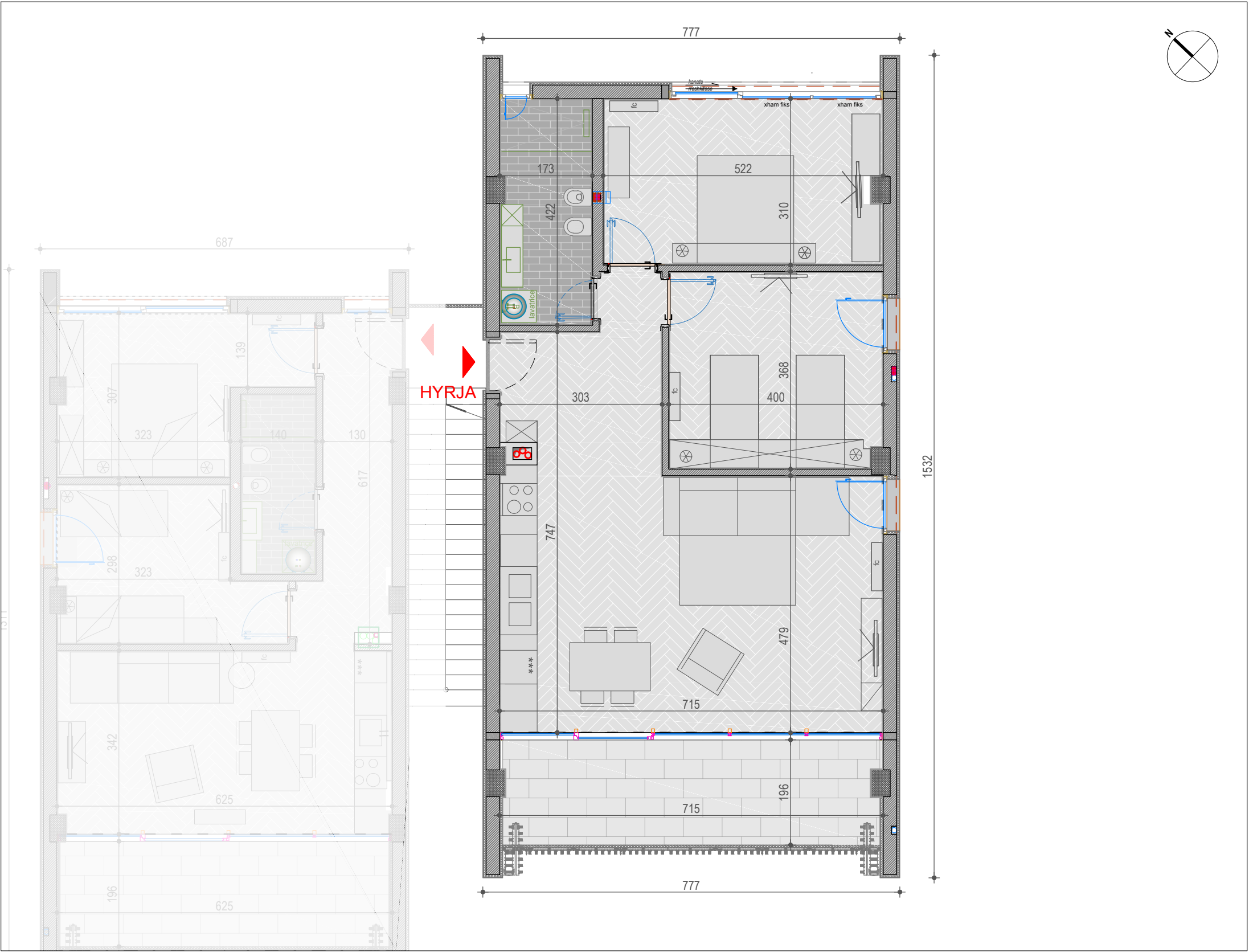
Planimetri Kati Përdhe
